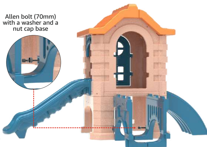
Subassembly (Step 10)
