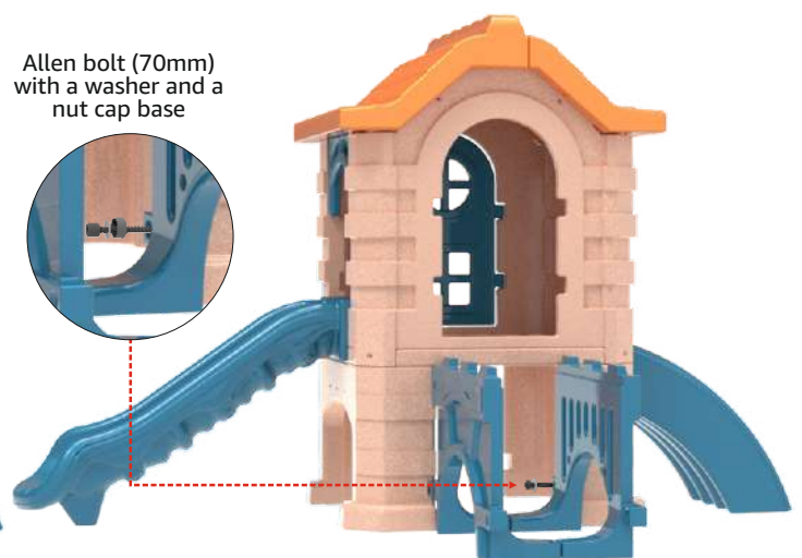
Subassembly (Step 10)
